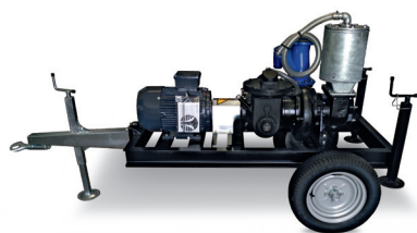
Elettropompa vuotoassistita
