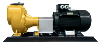
Electropompe auto-amorçante
