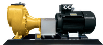
Elettropompa autoadescante
